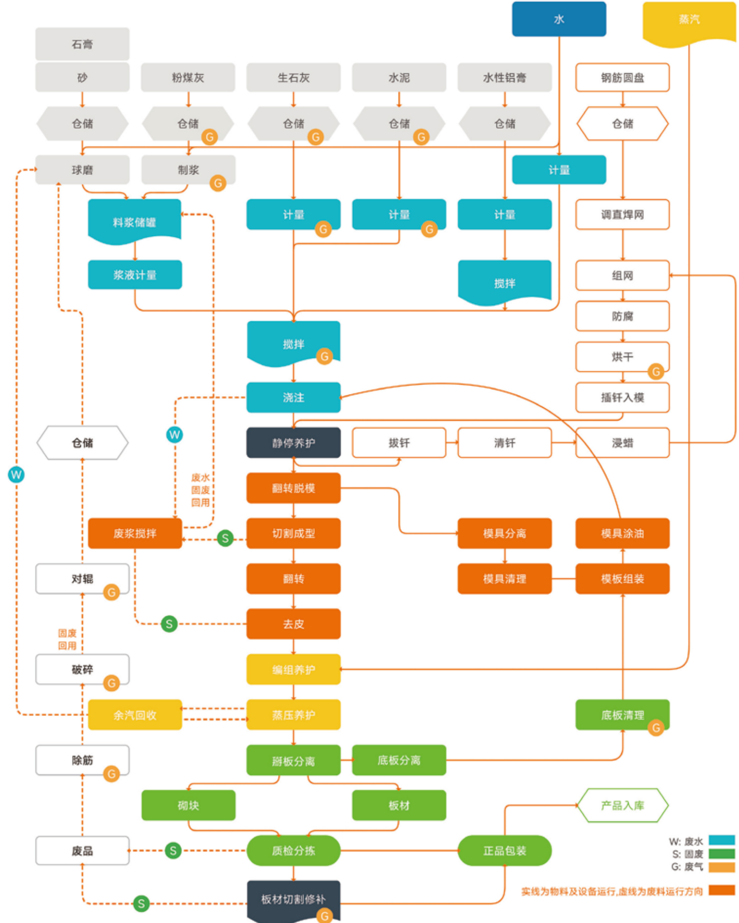
蒸压加气混凝土砌块/板材生产流程图
