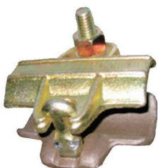
意式一半扣件 Italian Type Half Coupler 48.3mm 0.85kg
