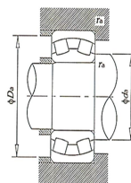
圆锥孔(1:12)20000K型
