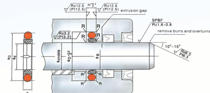
NO. 规格/d*H NO. 规格/d*H NO. 规格/d*H 20*3.2 65*6.3 190*6.3 25*3.2 70*4.2 200*8.1 28*3.2 70*6.3 210*8.1 30*3.2 75*4.2 220*8.1 32*3.2 75*6.3 230*8.1 35*3.2 80*4.2 240*8.1 20*4.2 80*6.3 250*8.1 22*4.2 85*6.3 260*8.1 25*4.2 90*6.3 270*8.1 28*4.2 100*6.3 280*8.1 30*4.2 105*6.3 290*8.1 32*4.2 110*6.3 300*8.1 35*4.2 115*6.3 310*8.1 36*4.2 120*6.3 320*8.1 38*4.2 125*6.3 330*8.1 40*4.2 130*6.3 340*8.1 40*6.3 135*6.3 350*8.1 45*4.2 140*6.3 360*8.1 45*6.3 150*6 370*8.1 50*4.2 150*8.1 380*8.1 50*6.3 155*6.3 400*8.1 55*4.2 160*6.3 420*8.1 55*6.3 160*8.1 440*8.1 60*4.2 170*6.3 450*8.1 60*6.3 170*8.1 460*8.1 63*4.2 175*6.3 470*8.1 63*6.3 180*6.3 480*8.1 65*4.2 180*8.1 500*8.1
