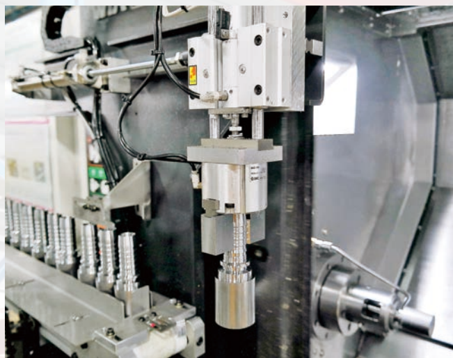
自动数控加工中心 Automatic CNC machining center
