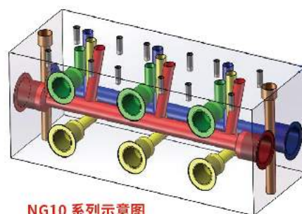
NG10 系列示意图
