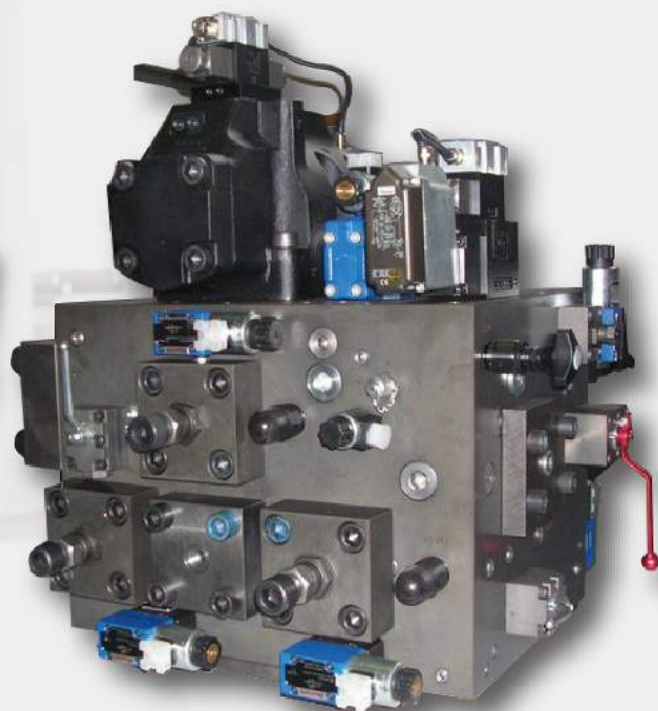
► 系统阀组 System valve group
