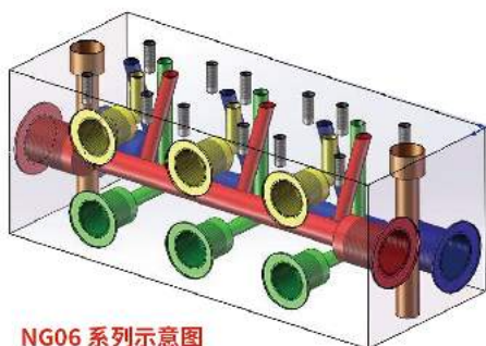
NG06 系列示意图
