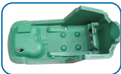
洗地机模具（下模）
