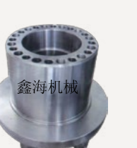
行星架 Planet Carrier
