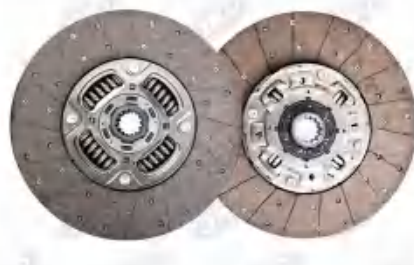
规格:430*14T*48 车型:三菱51JK
