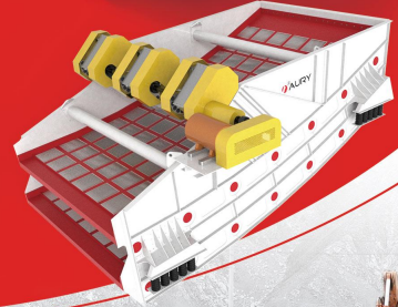
香蕉筛-双层
