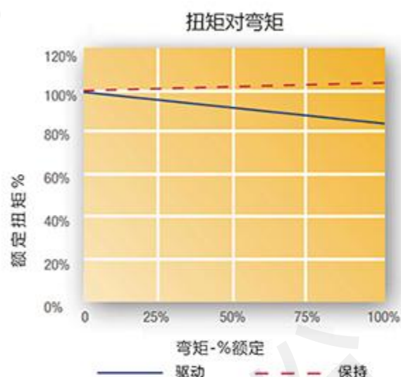
弯矩扭矩关系曲线
