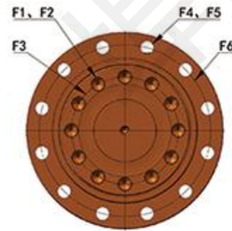
输出法兰
