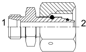
直通接头
