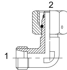
90°弯头
