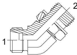
45°弯头
