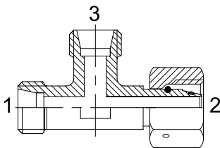
三通接头
