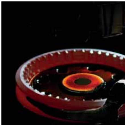
➤ Tempra a tampono. Plug quenching.
