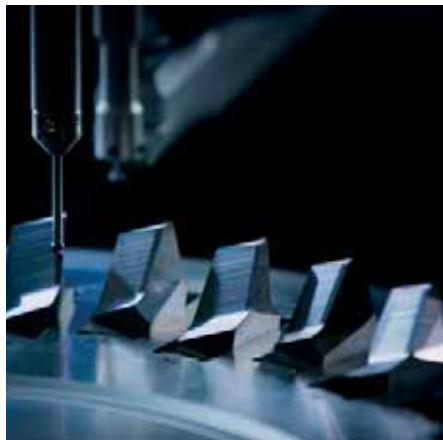
➤ Controllo posizionamento lame. Cutter positioning check.
