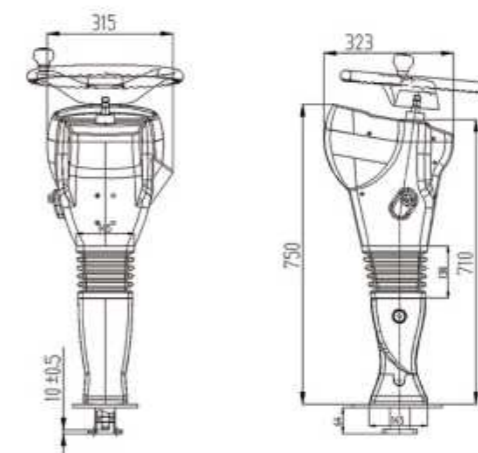
BHQ303/BHG303 适用：装载机等小型铲运工程机械
