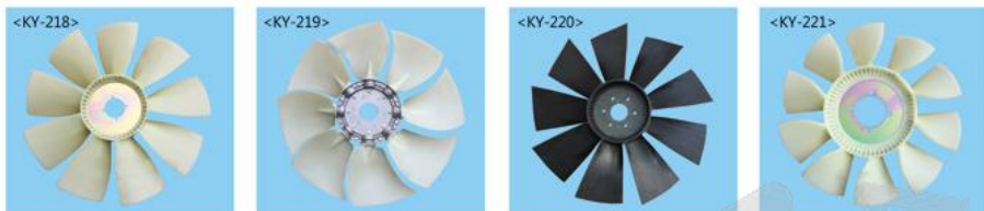
<KY-218> 沃尔沃210 240 750-82-96-4T9 710-82-96-4T9 <KY-219> 沃尔沃-770-76-134-6T8 <KY-220> 沃尔沃 360B 460B-750-76-134 <KY-221> 挖掘机多用可改装-460-86-103
