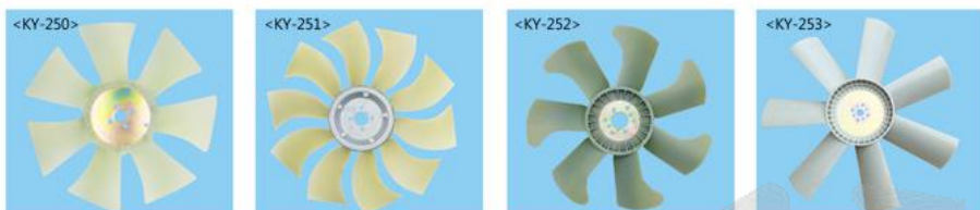
<KY-250> 洋马4TNV94 沃尔沃55-460-28-52-4T7 <KY-251> 徐工80-505-36-58-10 <KY-252> 小松老款4D95-550-50-75-89 <KY-253> 小松380
