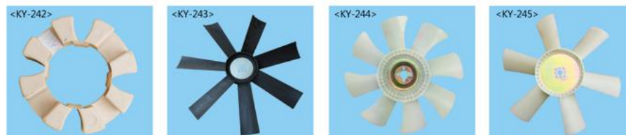
<KY-242> 连接胶 (2) <KY-243> 康明斯反吹直径1000mm <KY-244> 卡特加藤250 S4F4N40-430-30-50-4T8 <KY-245> 现代290-6BT5.9康明斯 660-25-50-60
