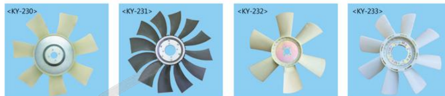
<KY-230> 三一挖掘机75 4JG1-480-34-56-4T7 <KY-231> 三一 徐工 柳工-560-75-96-4T12 <KY-232> 日立200-5 -720-178-215 <KY-233> 日立200-1-2-3 6BD1 600-108-128-48
