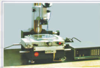
高精度万能工具显微镜 High Accuracy Universal Tool Microscope
