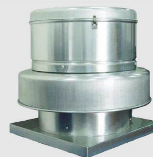
DWL屋顶离心排风机 DWL Rooftop Centrifugal Exhaust Fan
