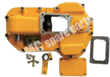
Имя Тормозная лента в сборе Name Brake Ass'y Nombre Conjunto de Freno Suitable for Bulldozers: SHANTUI / KOMATSU / ZOOMLION / HBXG / XCMG
