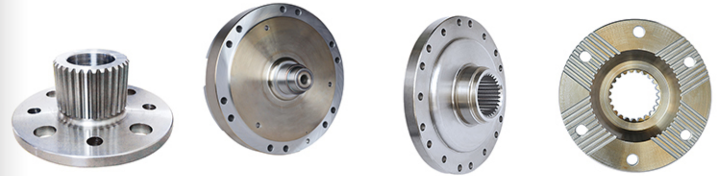
50型直接档连接盘 Direct gear connection platen type 50 直接档油缸 Direct gear cylinder 50型直接档受压盘 Direct Gear Pressure Platen type50 端面齿输入法兰 End-face ring input flange
