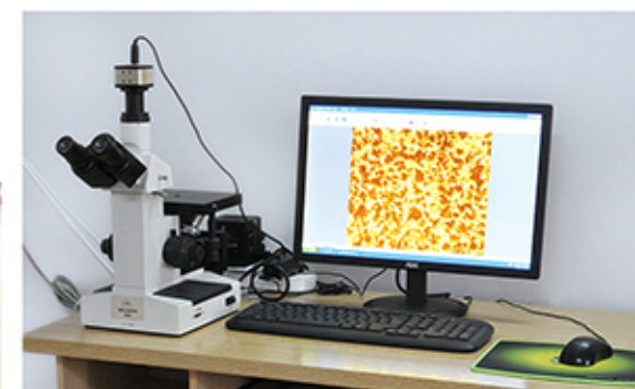
金相分析仪
