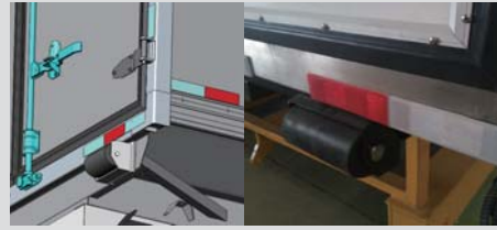
新型专利防撞滚轮 防撞滚轮设计，有效的保护厢体和厢内货物安全！
